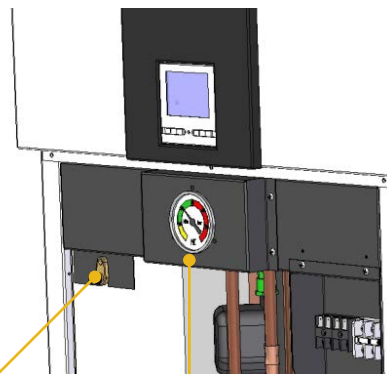
Manometer
